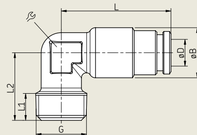
Kniestück
