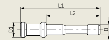
Verschlussstift
