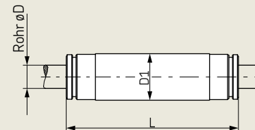
Rohrverbinder
