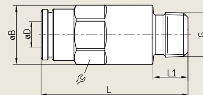
Rückschlagventil
