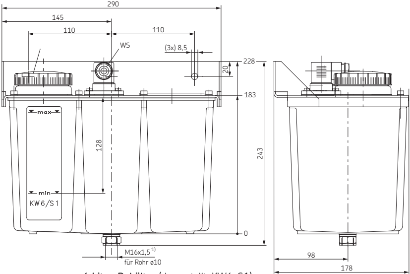
6 Liter-Behälter (dargestellt: KW6-S1)
