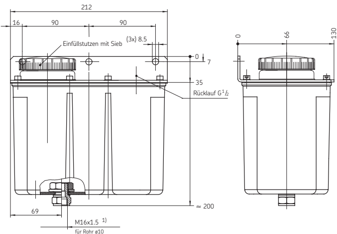
3 Liter-Behälter (dargestellt: K3-S2)
