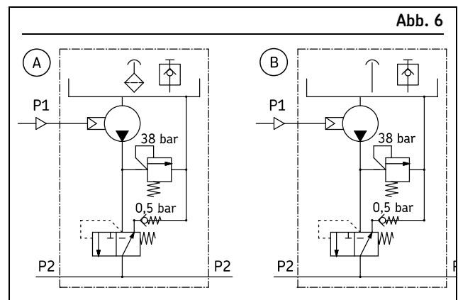
Hydraulischer Schaltplan der pneumatisch betriebenen Einkolbenpumpe ACP (A: Öl; B: Fließfett)
