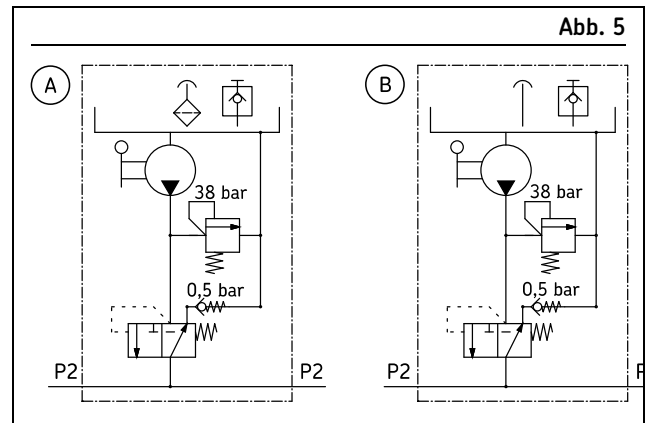
Hydraulischer Schaltplan der handbetriebenen Einkolbenpumpe MCP (A: Öl; B: Fließfett)
