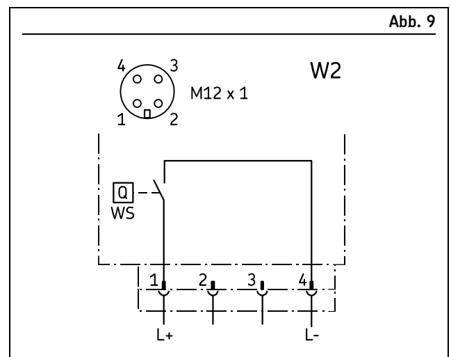
Rundsteckverbinder für den Schwimmerschalter (Darstellung: Schwimmerschalter bei leerem Behälter)
